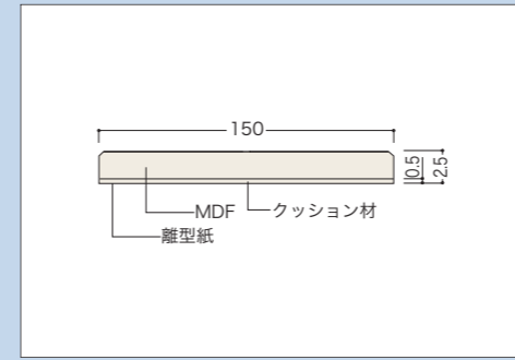
■断面図(mm)
